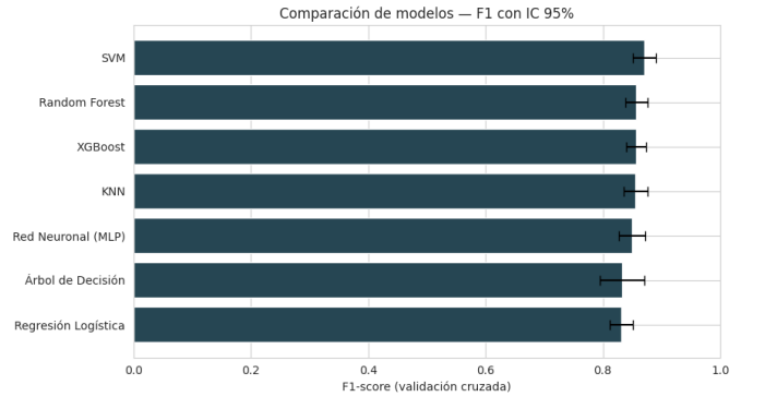
Figura 2. Comparación de modelos por F_1 en validación cruzada con intervalos de confianza al 95 %. El solapamiento de los intervalos indica que las diferencias entre modelos no son estadísticamente significativas.
