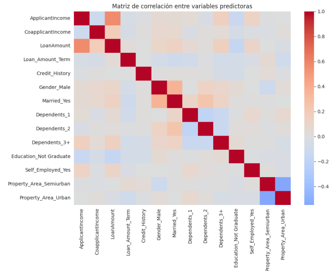
Figura 6. Matriz de correlación entre variables predictoras. La ausencia de correlaciones fuertes indica baja redundancia entre variables.
